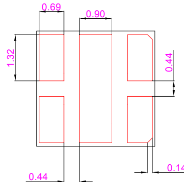
推荐钢网尺寸
