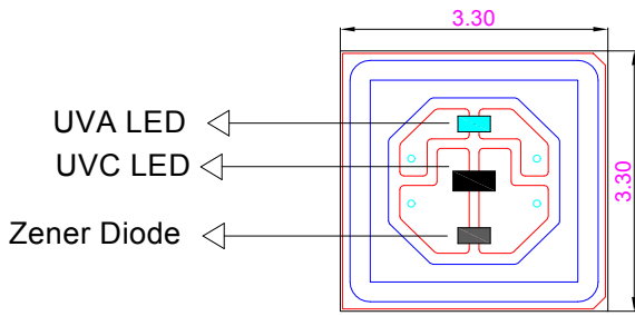
俯视图
