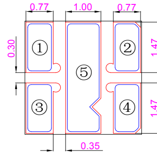
底部焊盘 (透视图)
