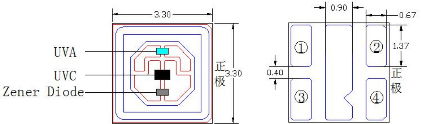
底部焊盘 (透视图)
