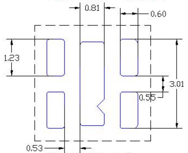
推荐钢网尺寸
