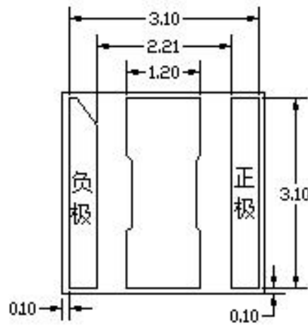
底部焊盘 (透视图)
