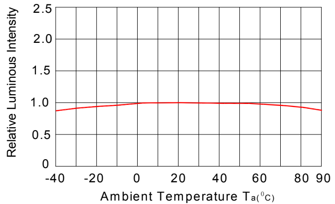
Fig.4 相对亮度 Vs. 环境温度
