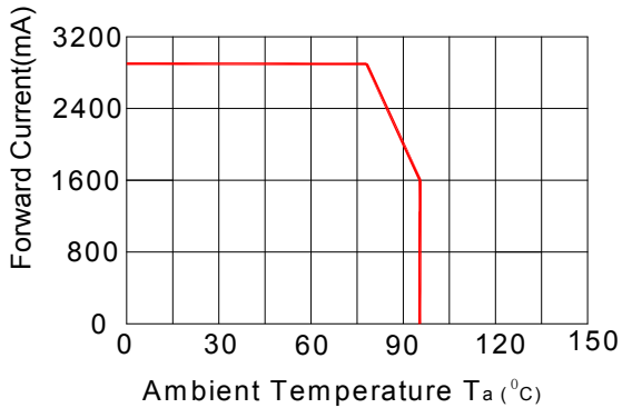
Fig.3 正向电流 Vs. 环境温度
