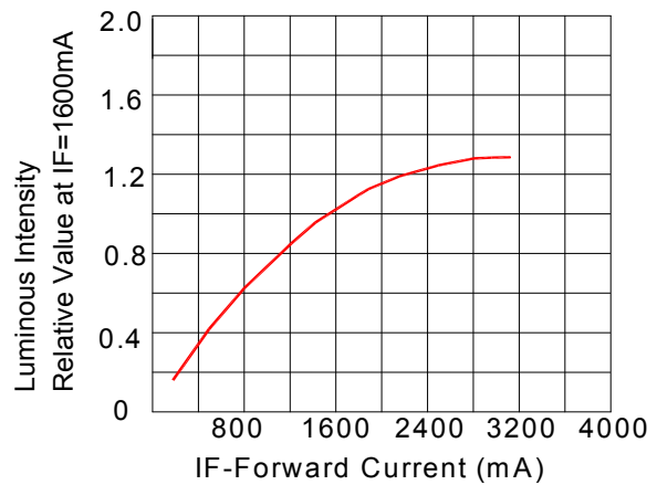
Fig.2 相对亮度 Vs. 正向电流
