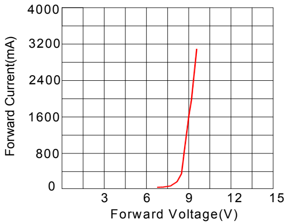
Fig.1 正向电流 Vs. 正向电压
