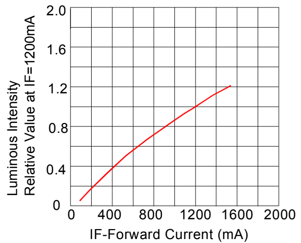
Fig.2 相对亮度 Vs. 正向电流
