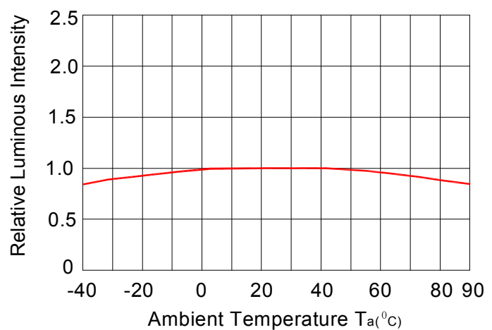
Fig.4 相对亮度 Vs. 环境温度
