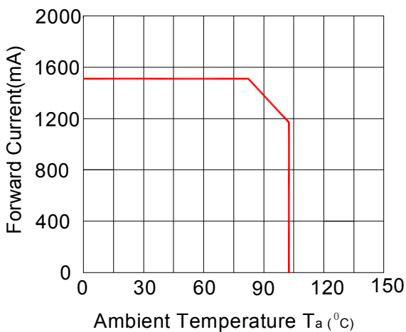
Fig.3 正向电流 Vs. 环境温度
