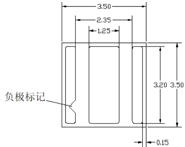
底部焊盘 (透视图)
