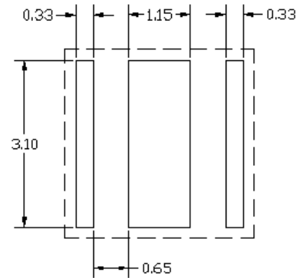
推荐钢网尺寸
