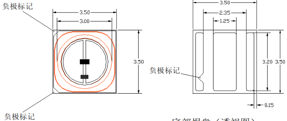
底部焊盘 (透视图)
