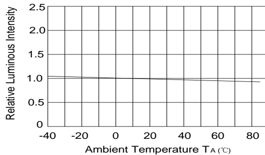
Fig.4 相对亮度 Vs. 环境温度
