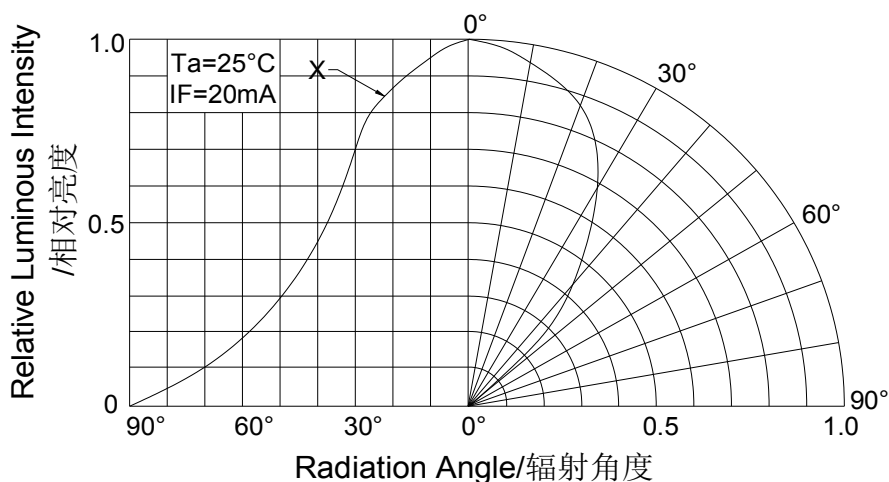
DIRECTIVITY/指向角度
