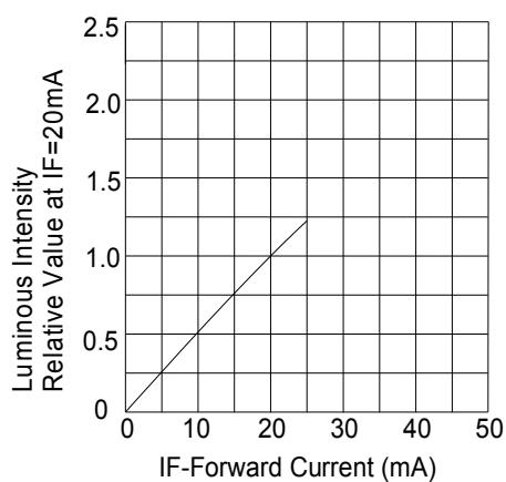
Fig.2 相对亮度 Vs. 正向电流
