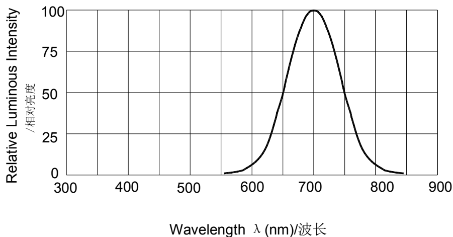
Fig.5 辐射强度 Vs. 波长
