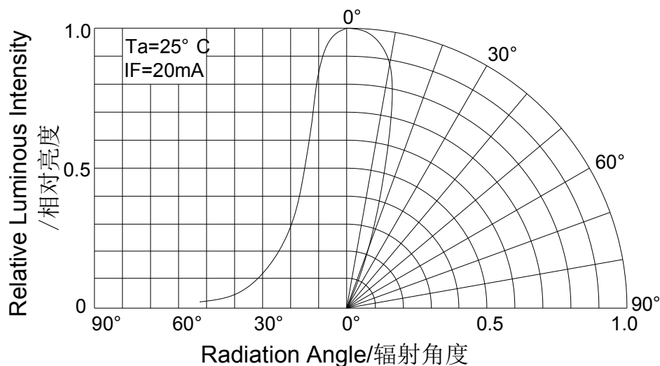
DIRECTIVITY/指向特性
