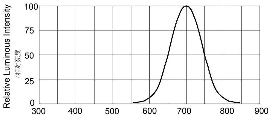
Fig.5 辐射强度 Vs. 波长
