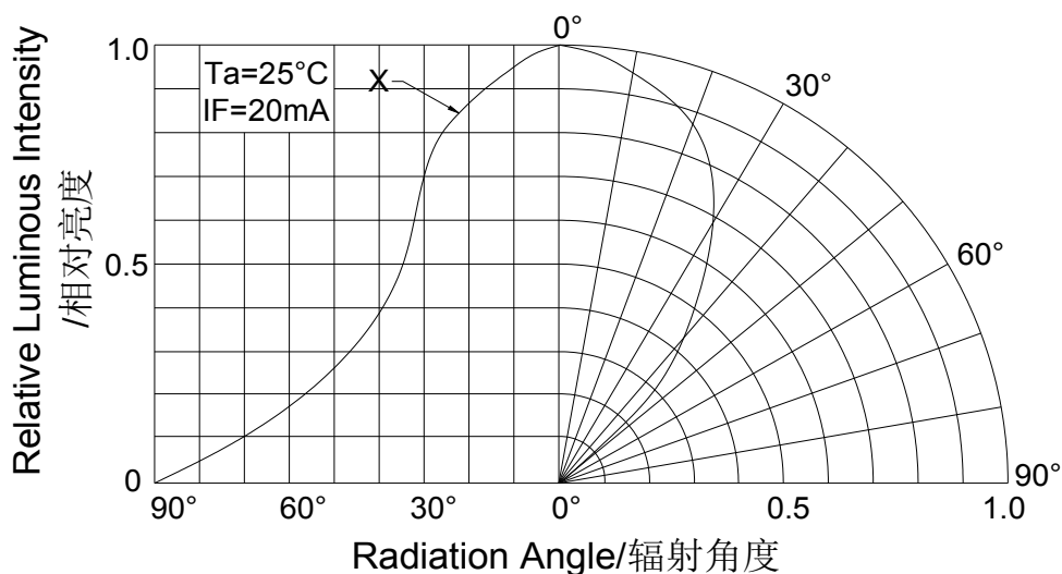
DIRECTIVITY/指向角度
