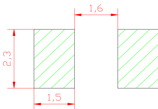
参考焊盘尺寸
