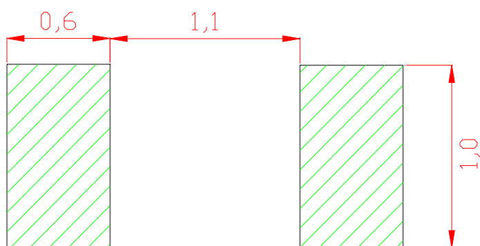
参考焊盘尺寸
